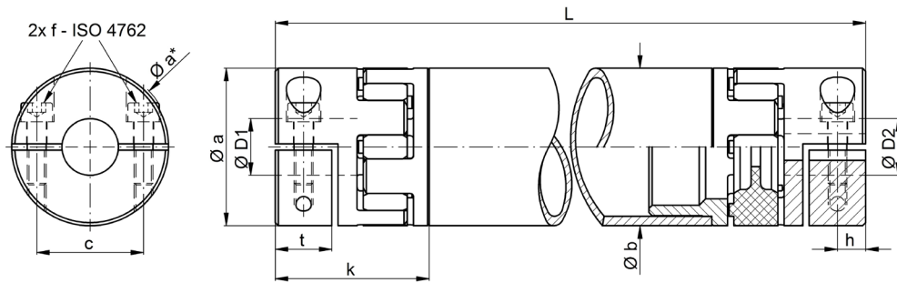
Distanzkupplung EWLH
