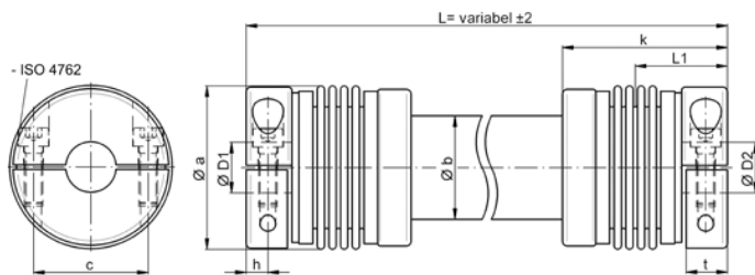
Distanzkupplung EWLC
