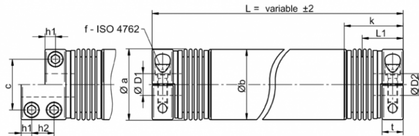
Distanzkupplung EWLM
